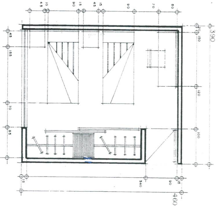
RECAMARA PARA DOS PERSONAS
