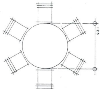
MESA REDONDA PARA 6 PERSONAS
